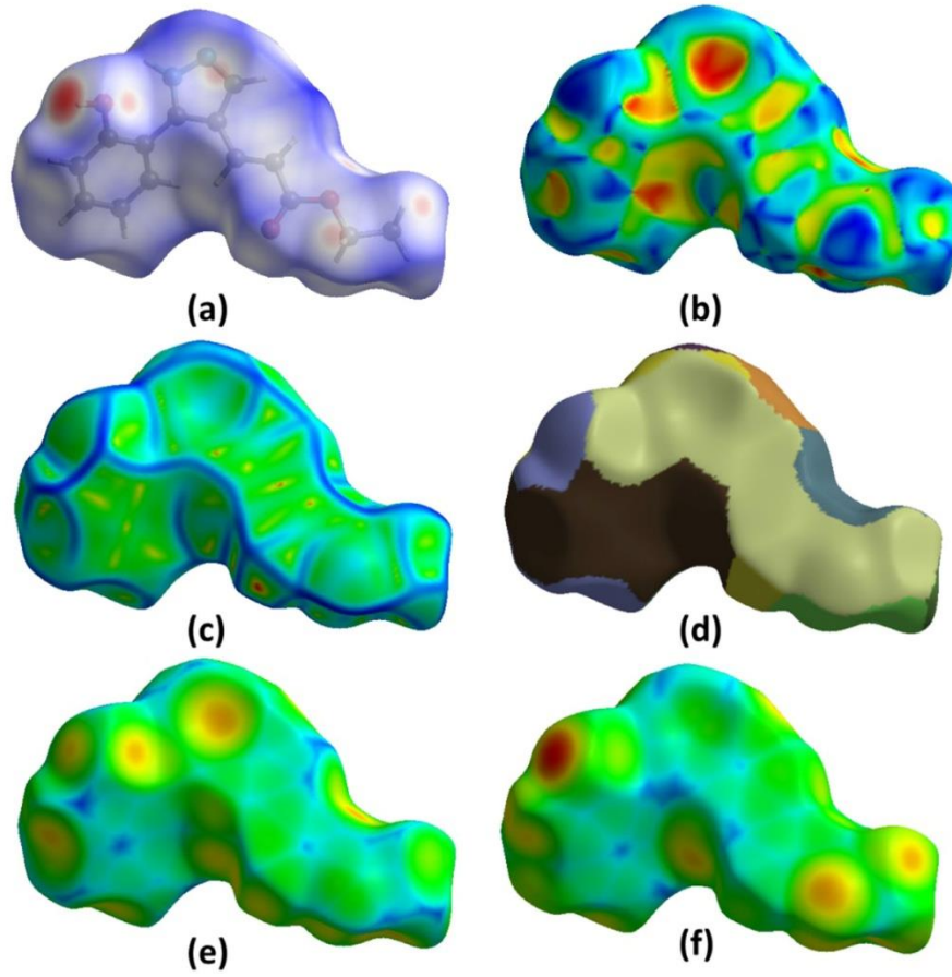
Resim 1.2. Bileşik 4 için Hirshfeld yüzey haritaları
